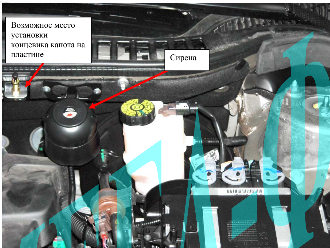
Рис. 6: Возможное место установки сирены и концевика капота.
