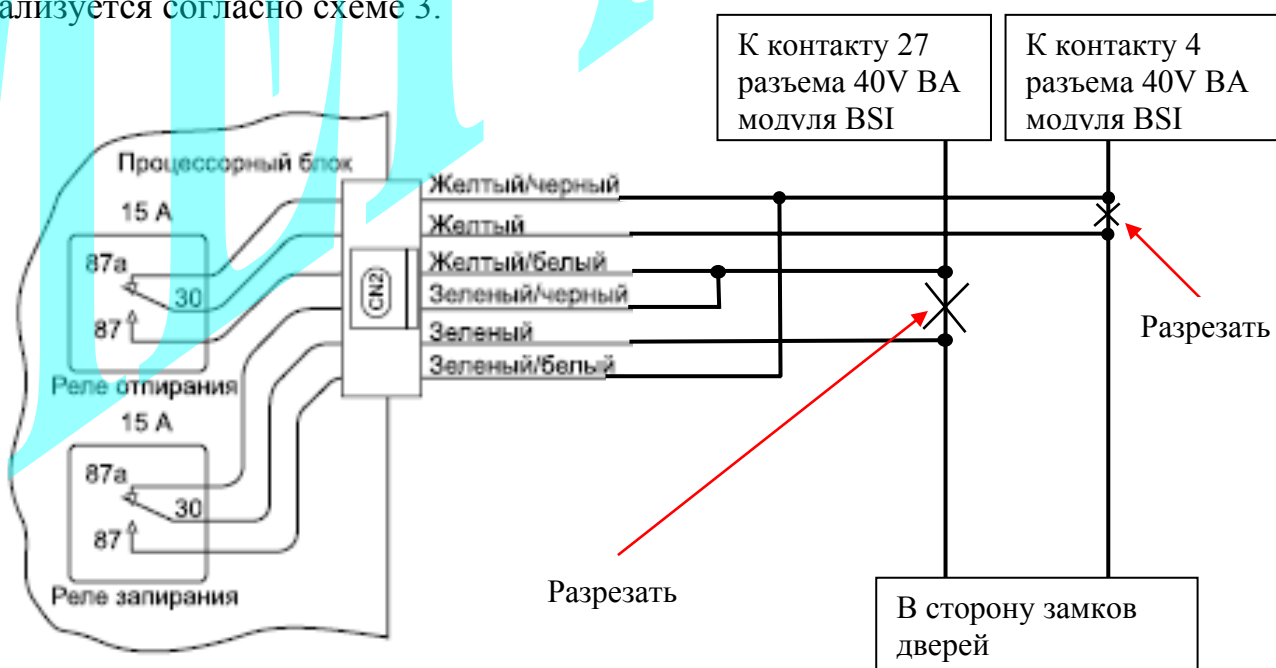
Схема 3: Подключение ЦЗ.
